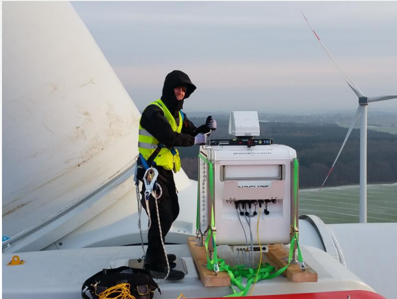
Ein ForWind-Wissenschaftler installiert das laser-optische Lidar-Messgerät zur Erfassung der Nachlaufströmung auf der Gondel einer Windenergieanlage der Firma eno energy. (Foto: Stephan Voß, ForWind)
